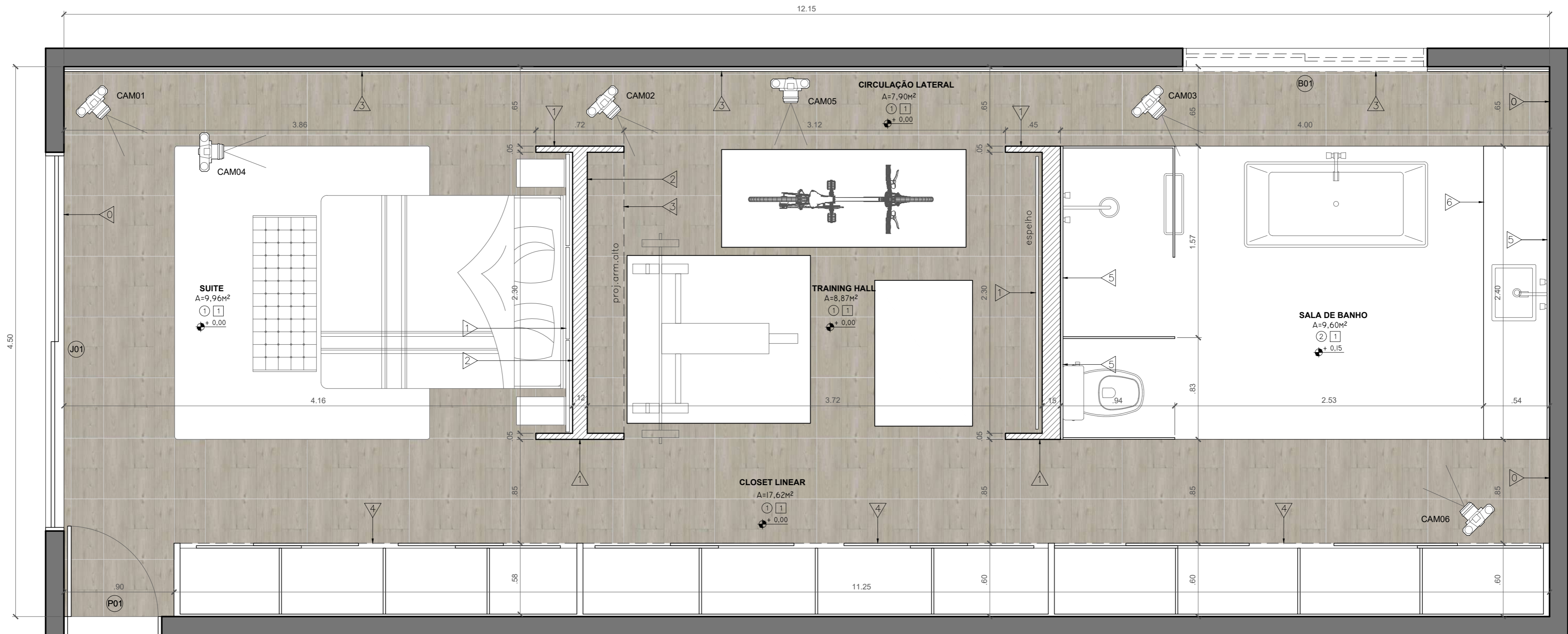
PLANTA BAIXA - Dormitório esc: 1/25
